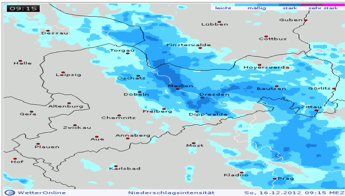
Schlechtwettergebiet über Dresden genau zu Beginn der DUR-Aktivität
