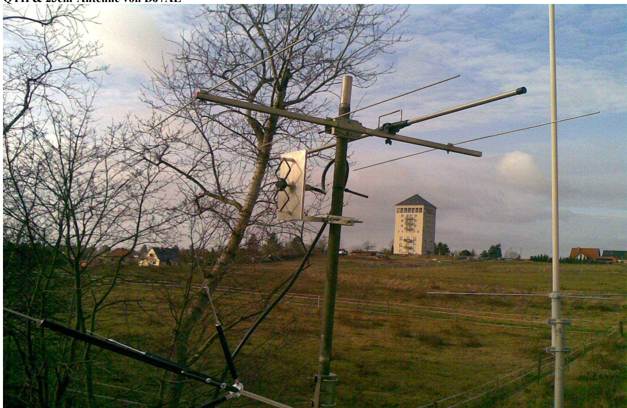
QTH & 23cm-Antenne von DJ7AL
